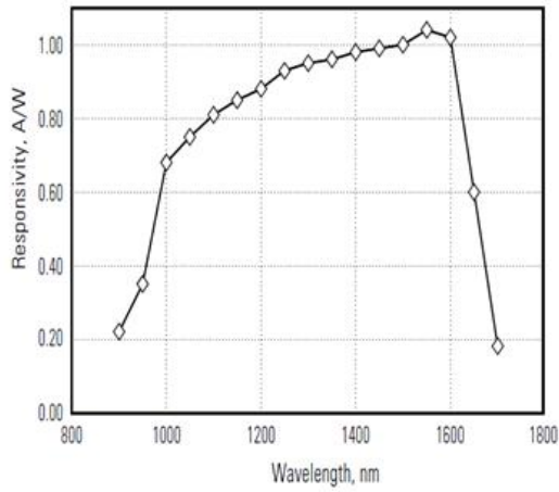
光谱响应
