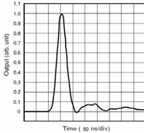
脉冲响应
